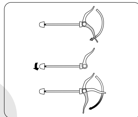
Apretar la tuerca de reglaje
