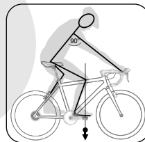
La rodilla debe estar posicionada por encima del eje del pedal delantero
